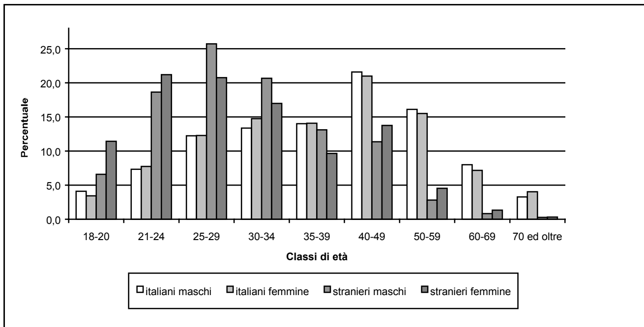
Grafico 1.1 - Composizione percentuale per sesso e classi di età dei denunciati italiani e stranieri - Anno 2001
