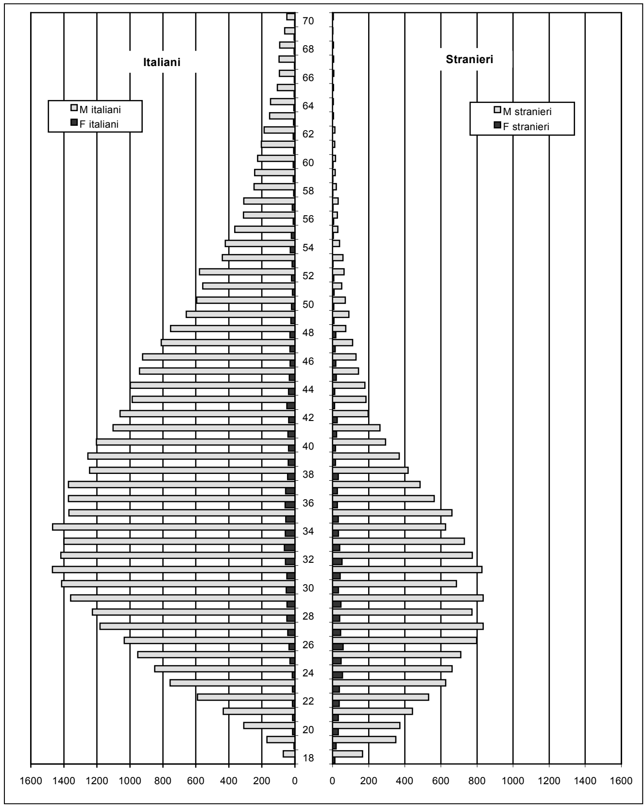
Grafico 4.2 - Popolazione detenuta al 31 Dicembre 2001: piramide delle età (valori assoluti)
